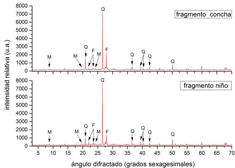
Figura n° 13.- Resultados del análisis de las piezas de terracota obtenidos por Difracción de Rayos X policristal. Permite identificar los principales compuestos cristalinos. SECYR© Proyecto El Saucedo.
